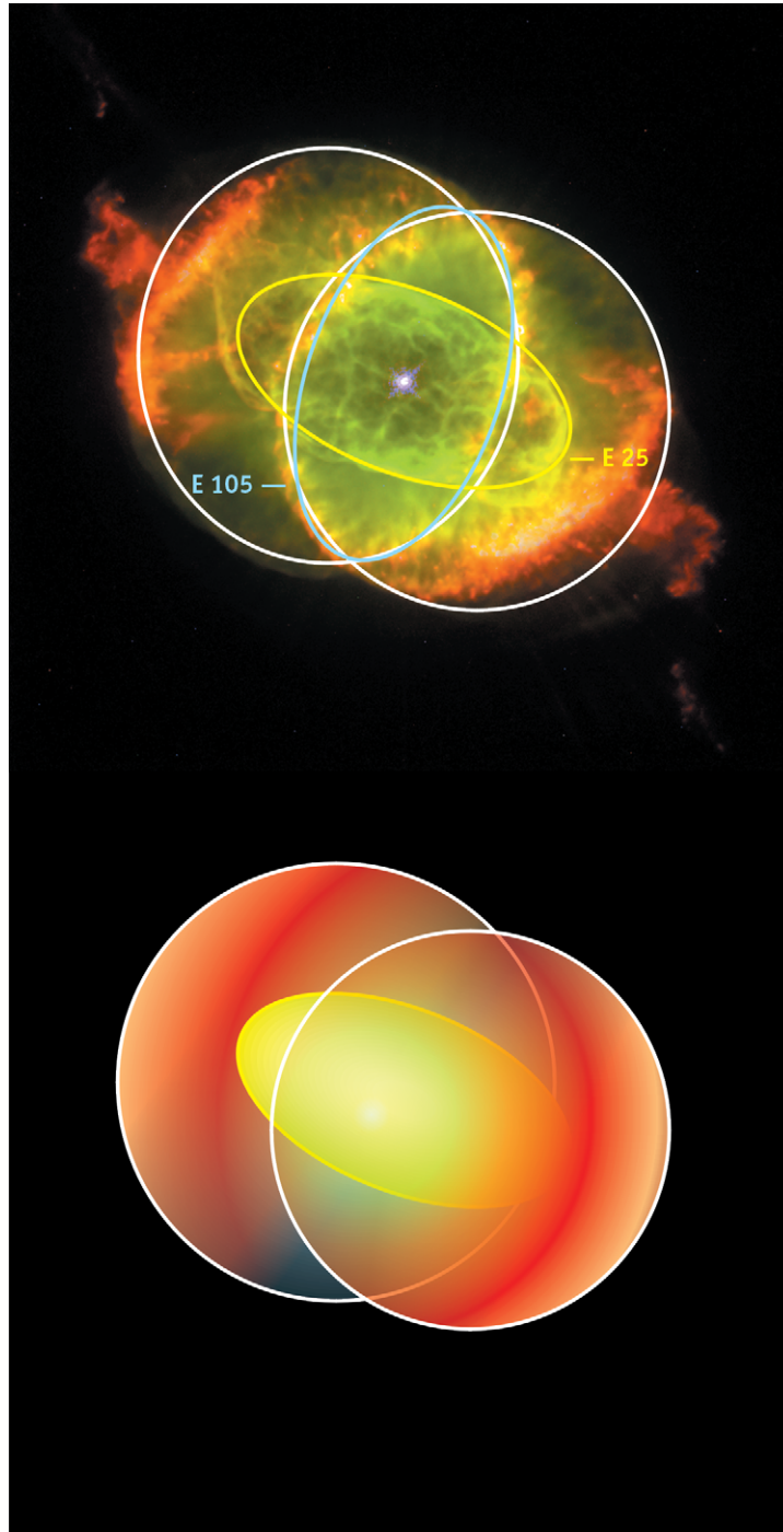
Figur 6: Geometrisk 3D-modell av Kattögennebulosan
