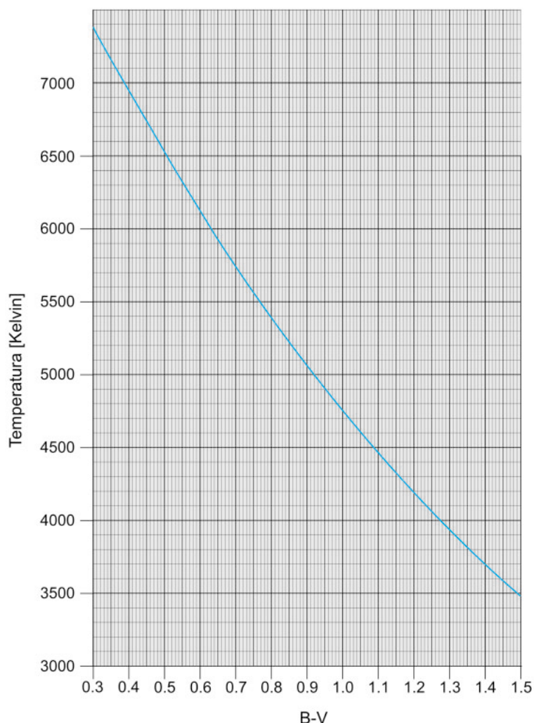
Figura 3: Temperatura superficial frente a índice de color B-V
