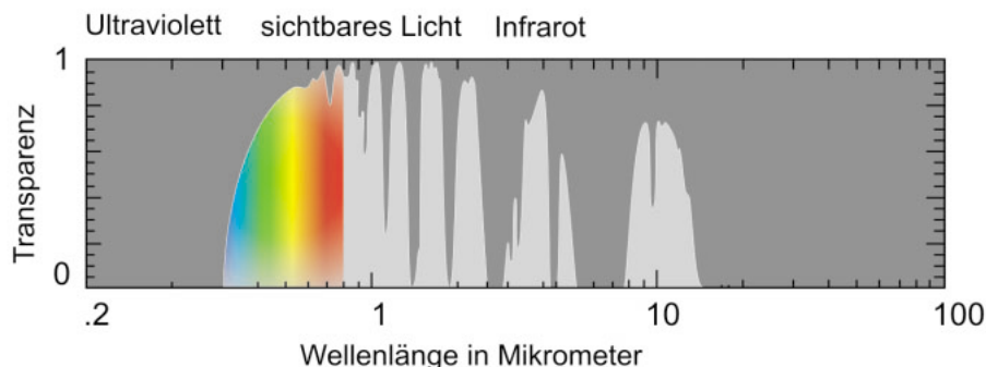
Abbildung 1: Absorption von Strahlung durch die Erdatmosphäre
