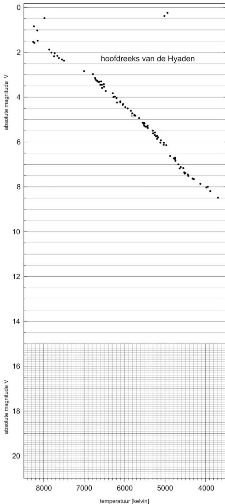
Figuur 11: H-R-diagram
